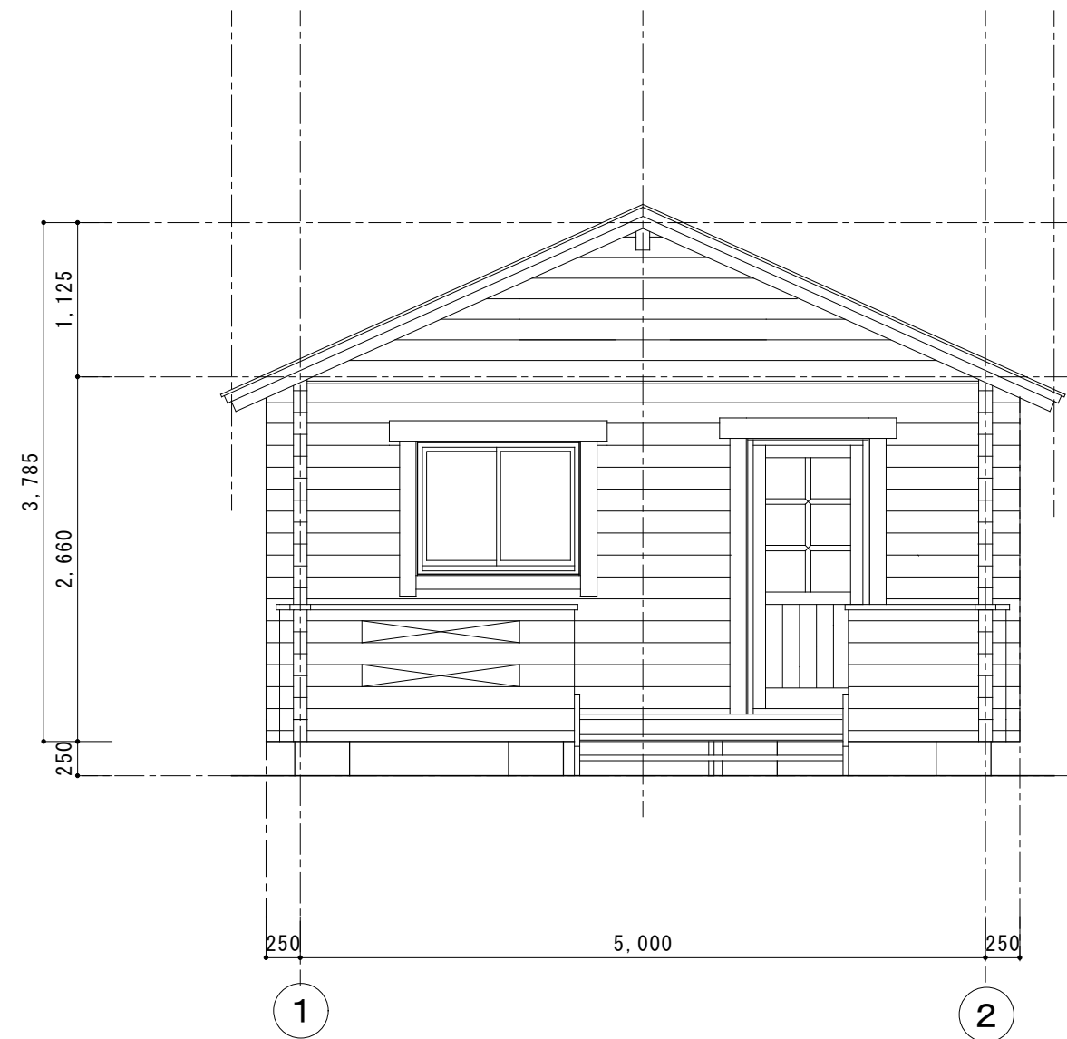
A通り立面図 1 / 50
