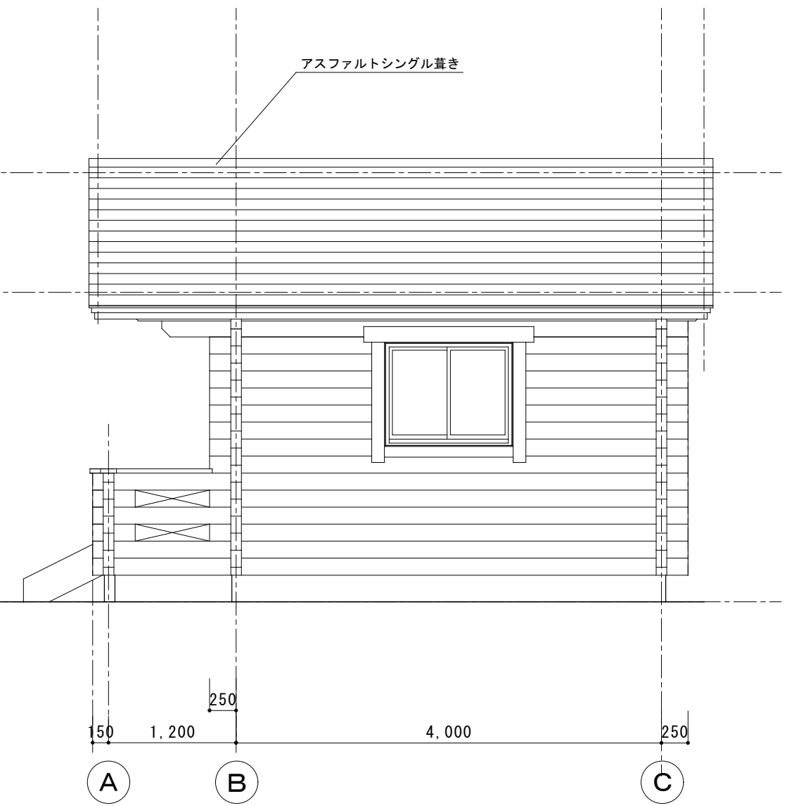
2通り立面図 1 / 50
