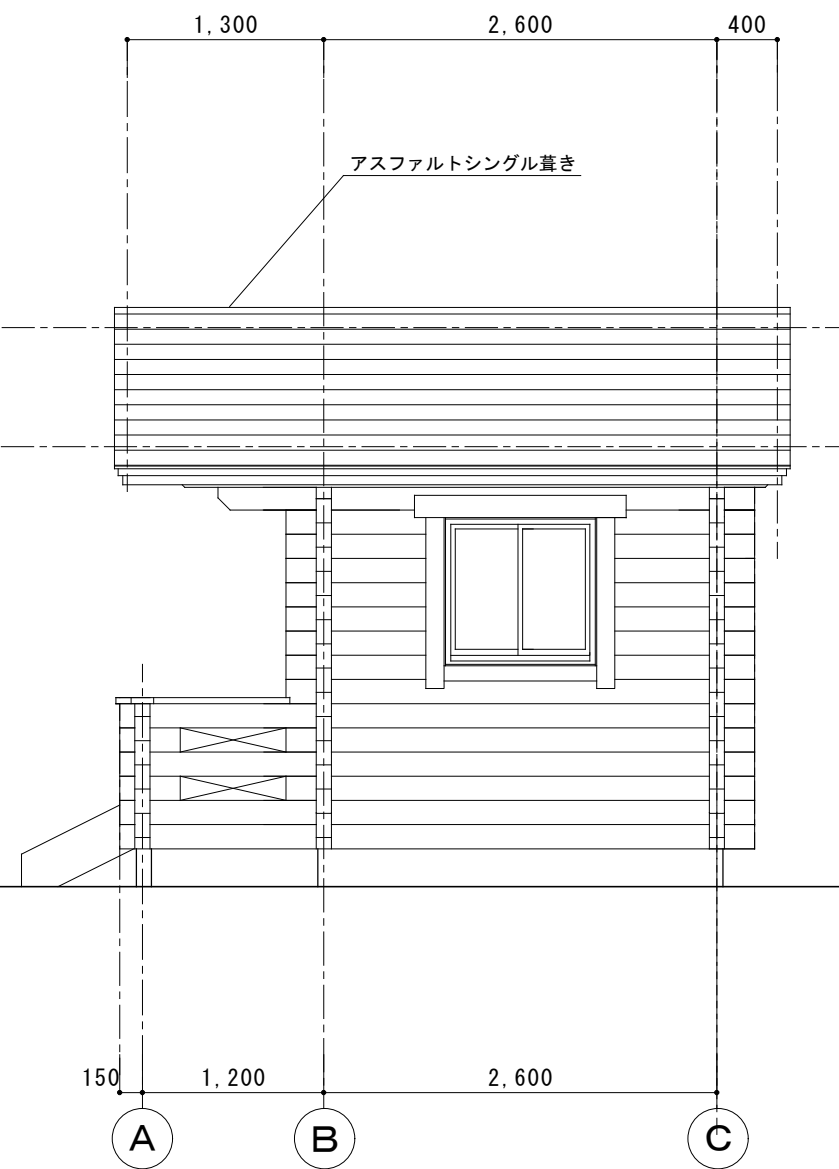
B 通り立面図 1 / 50
