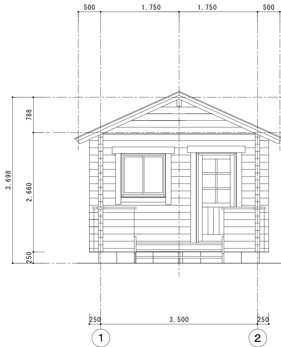
A 通り立面図 1 / 50
