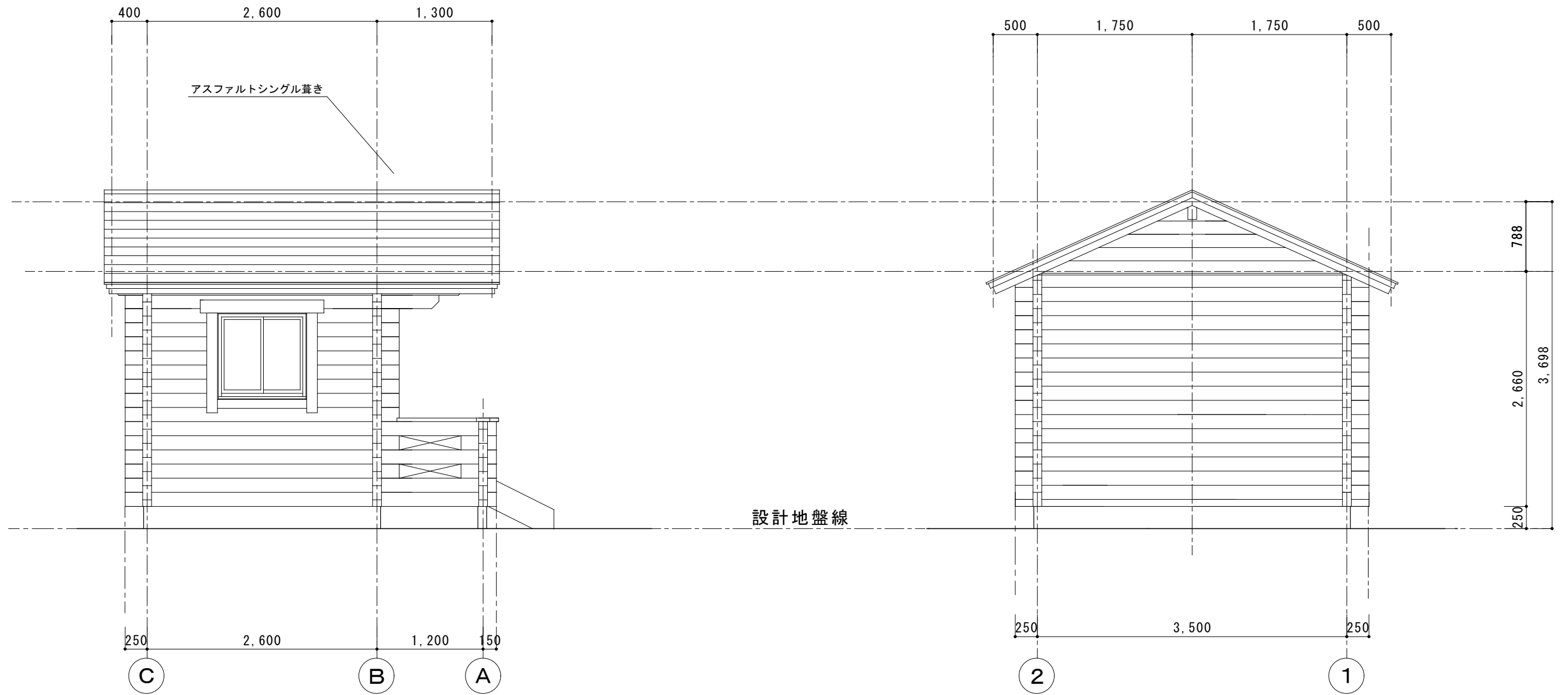
1通り立面図 1 / 50
